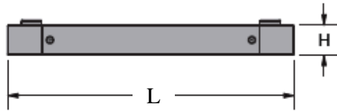
Vista frontale
