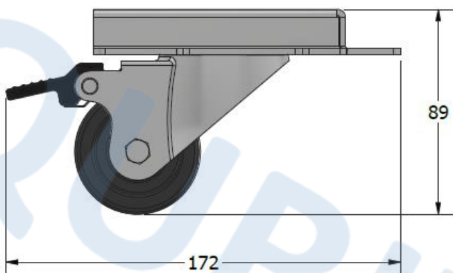
Vista frontale
