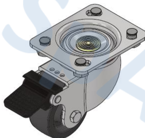
Vista isometrica
