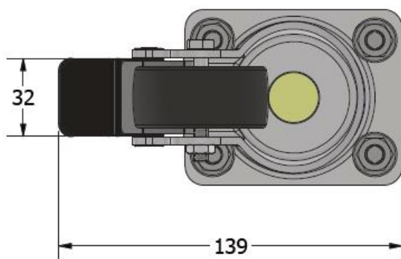
Vista dall'alto
