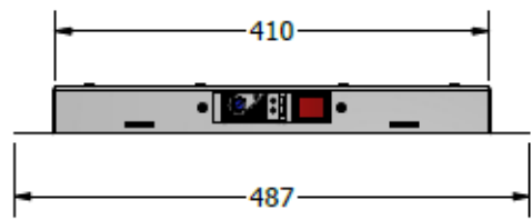
Vista frontale
