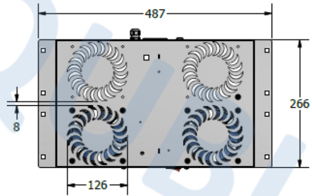
Vista dall'alto
