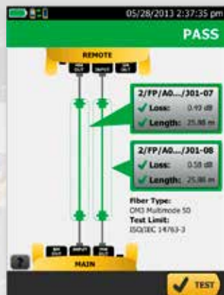
I dati completi sono visualizzati insieme al risultato del test. La linea tratteggiata mostra che cosa è incluso nella misurazione. Le finestre dei dettagli mostrano i risultati per ciascuna fibra testata.
